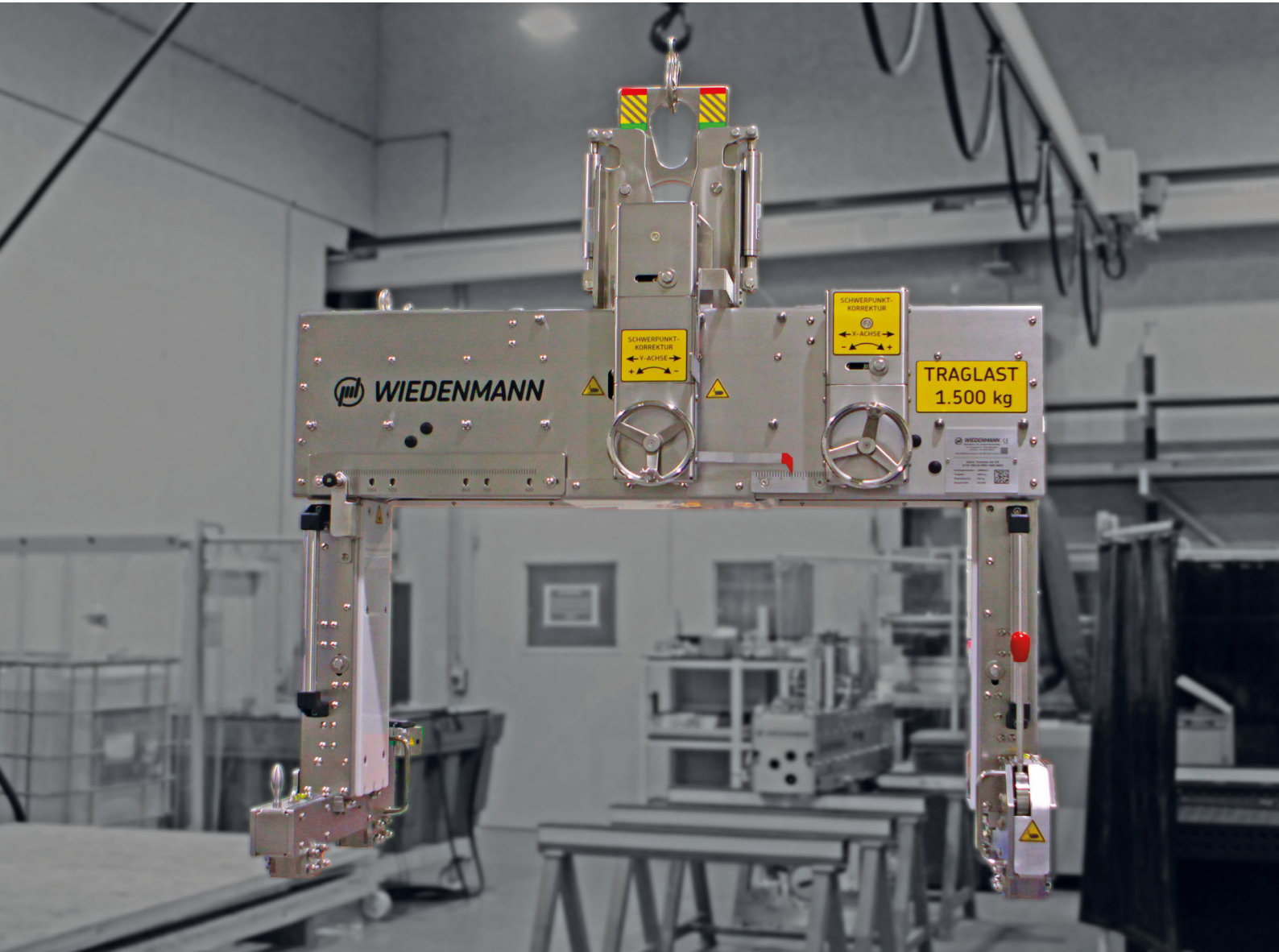
Mechanischer Hebegreifer aus nichtrostenden Edelstahl für Reinraumbetrieb ISO 6
