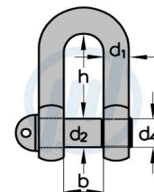
Form A mit Augbolzen
