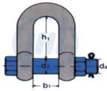
HC 1 gerade Form mit durchgehendem Bolzen, Mutter & Splint
