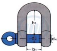
HA 1 gerade Form mit Schraubbolzen
