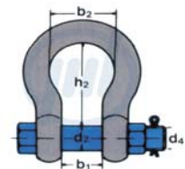
HC 2 geschweifte Form mit durchgehendem Bolzen, Mutter & Splint
